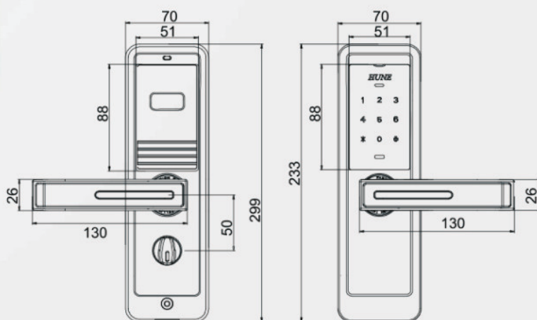
DIMENSION(mm)
